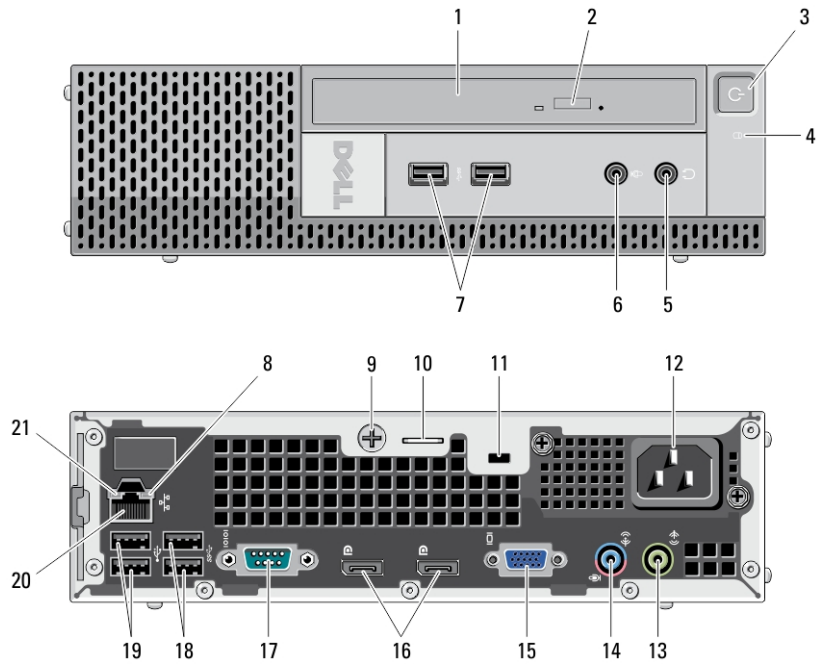
איור 5. מבט מלפנים ומאחור על מארז קטן במיוחד
