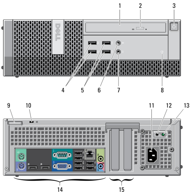
איור 3. מבט על הלוח האחורי של מחשב במארז קטן
