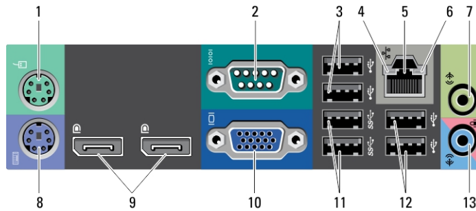
איור 4. תצוגת לוח אחורי של מארז קטן
